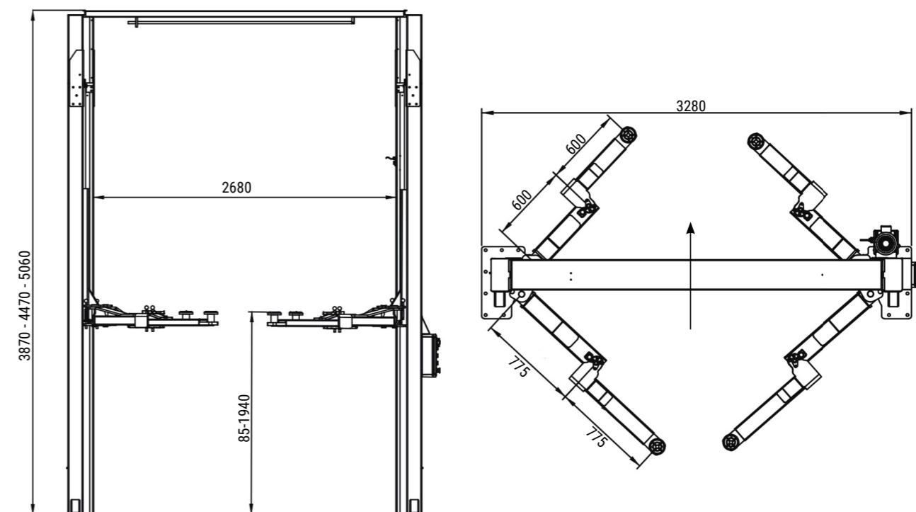
ROZŠÍRENIE KRÁTKYCH RAMIEN
