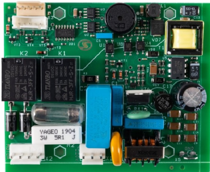
Doska pohonu SBMK 60 sputnik start , zdrojova doska
