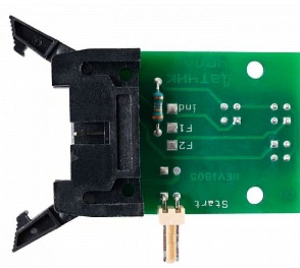
Snímač hriadeľa - CNY-70 s prídavným konektorom
